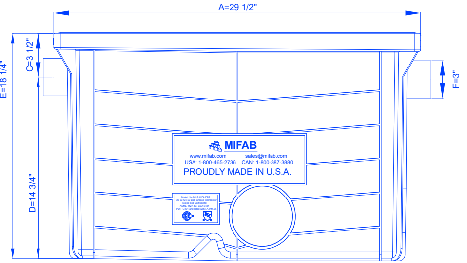
Elevation
