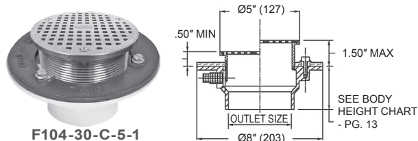
F104-30-C-5-1
