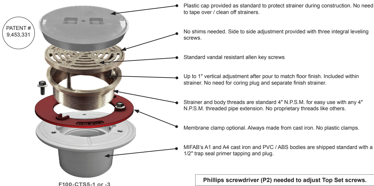
F100-CTS5-1 or -3
