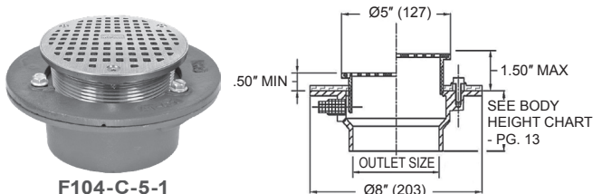
F104-C-5-1
