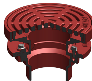
F324-4
