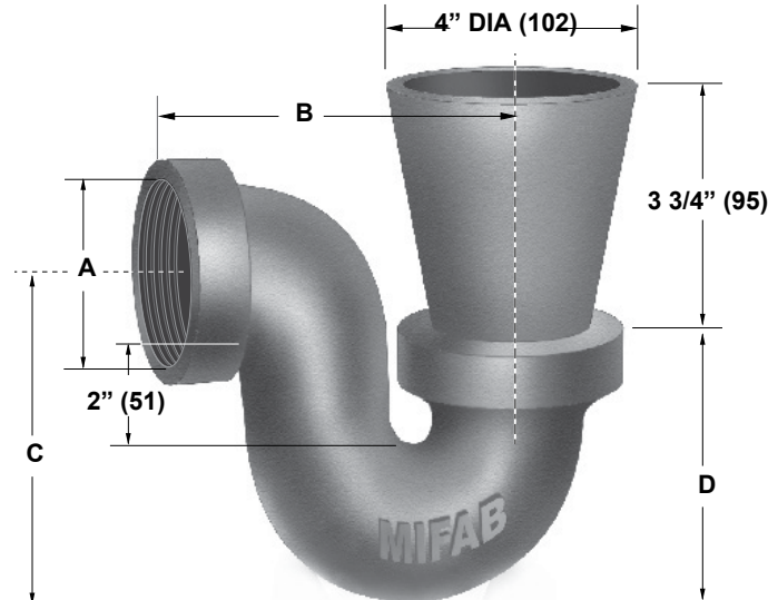
MI-940 DIMENSIONS
