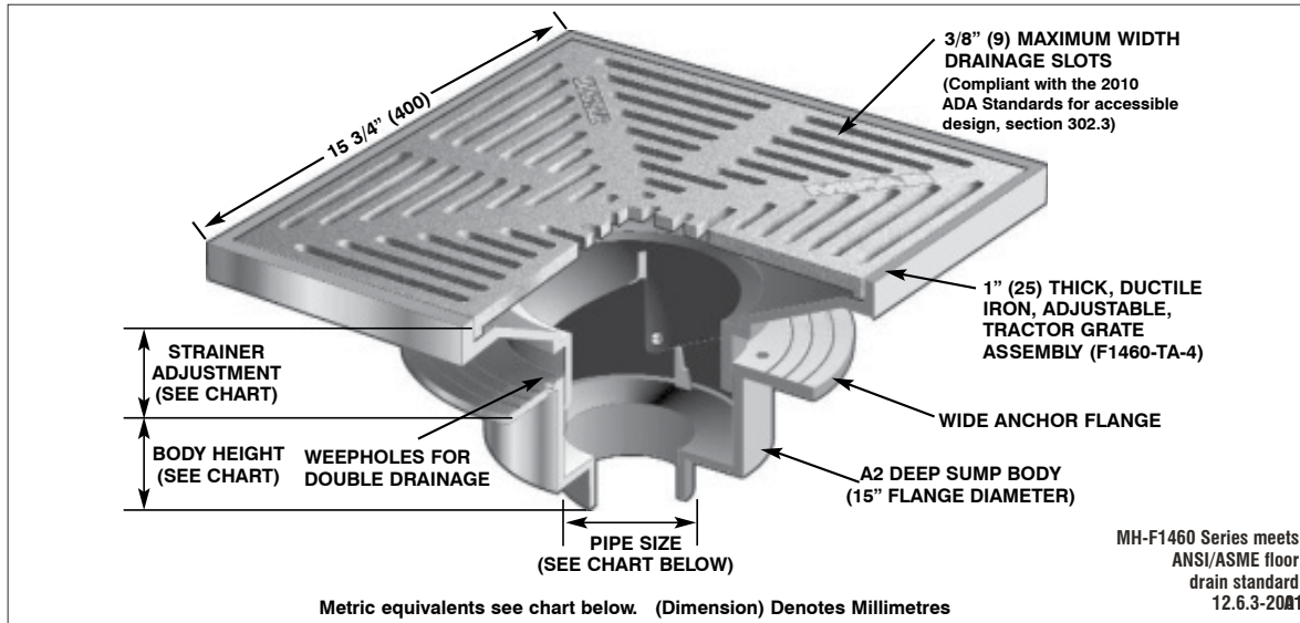
A2 Body
