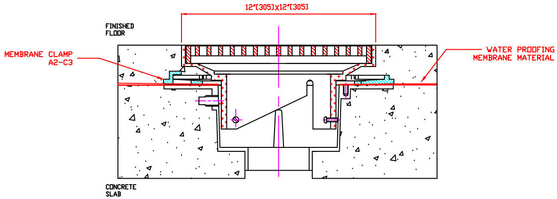
MEMBRANE INSTALL
